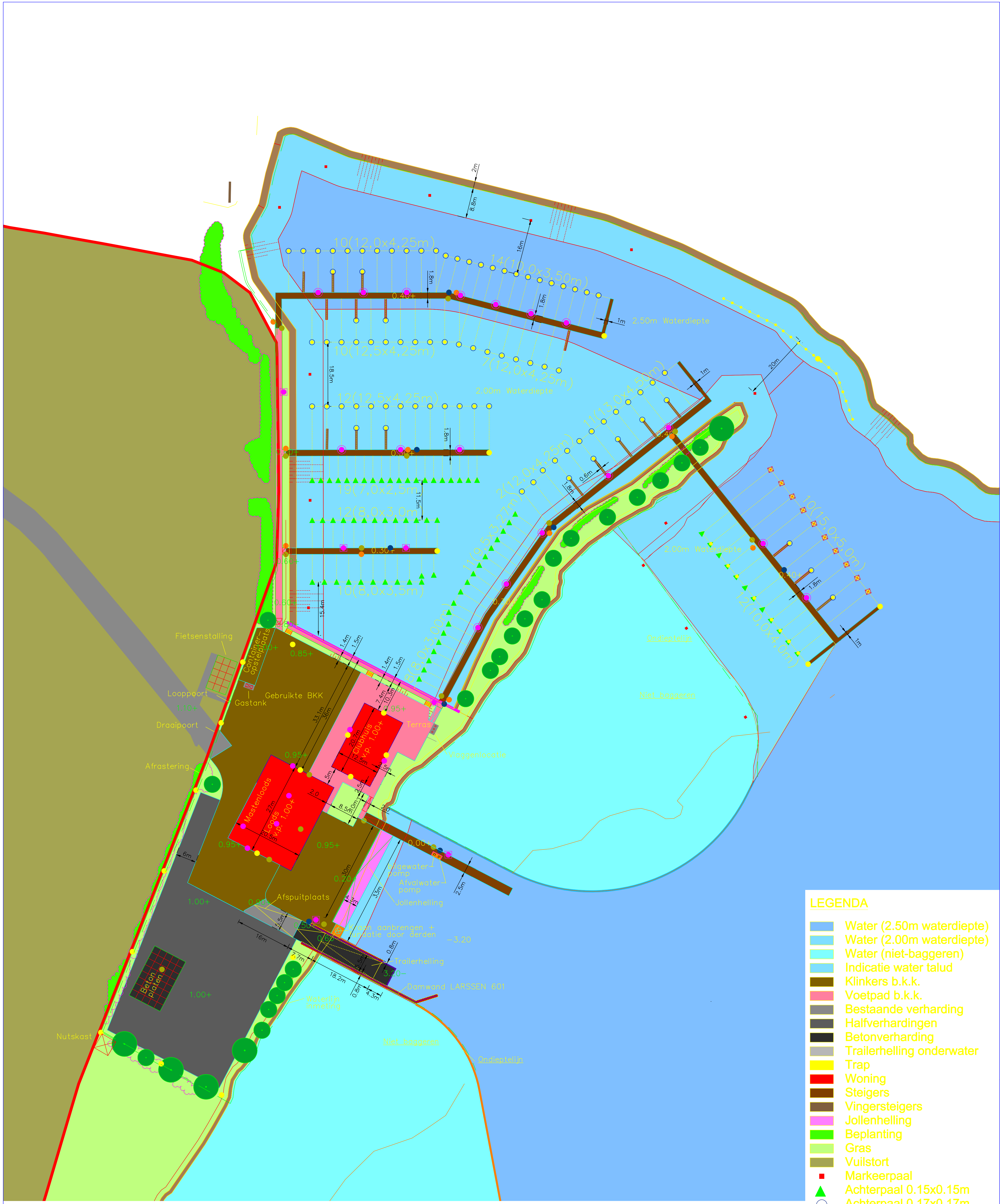
OVERZICHT SCHETSONTWERP JACHTHAVEN schaal 1:500
