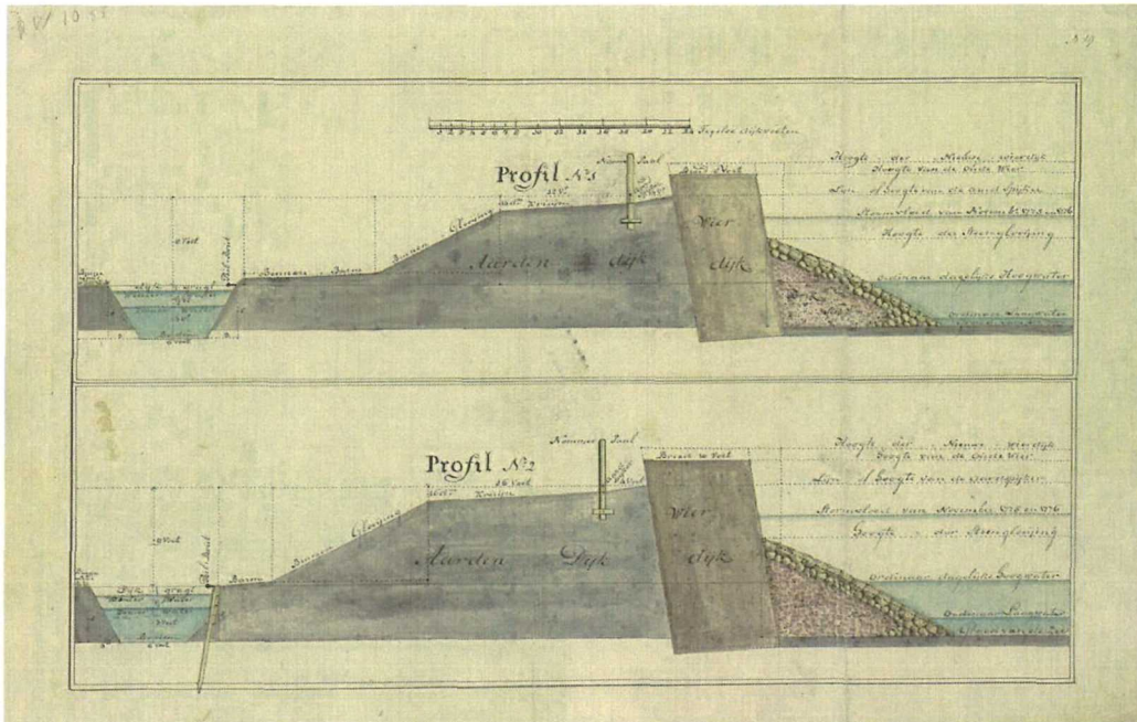
Technische tekening van Rijkswaterstaat: profiel van de dijk op Texel met aantekeningen van de hoogste stand van de stormvloed in november 1775 en 1776.
