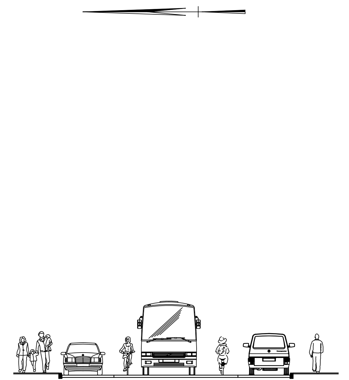
Principeprofiel 1 deel Italiëlaan - Belgiëlaan SCHAAL 1 : 100
