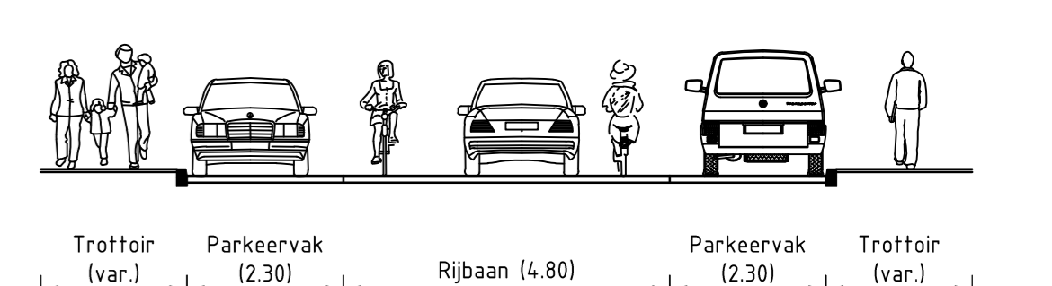
Principeprofiel 2 deel Vilniusstraat - Italiëlaan SCHAAL 1 : 100
