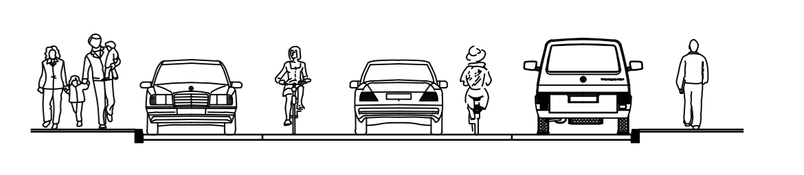
Principeprofiel 2 deel Vilniusstraat - Italiëlaan SCHAAI 1 : 100
