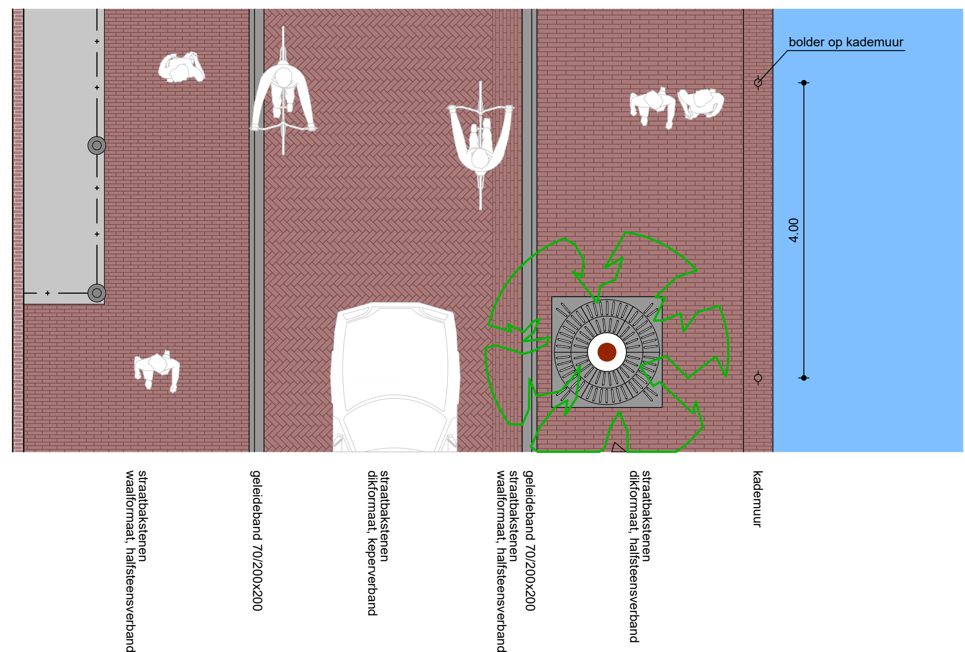
Principeprofiel B-B (geen parkeren)
