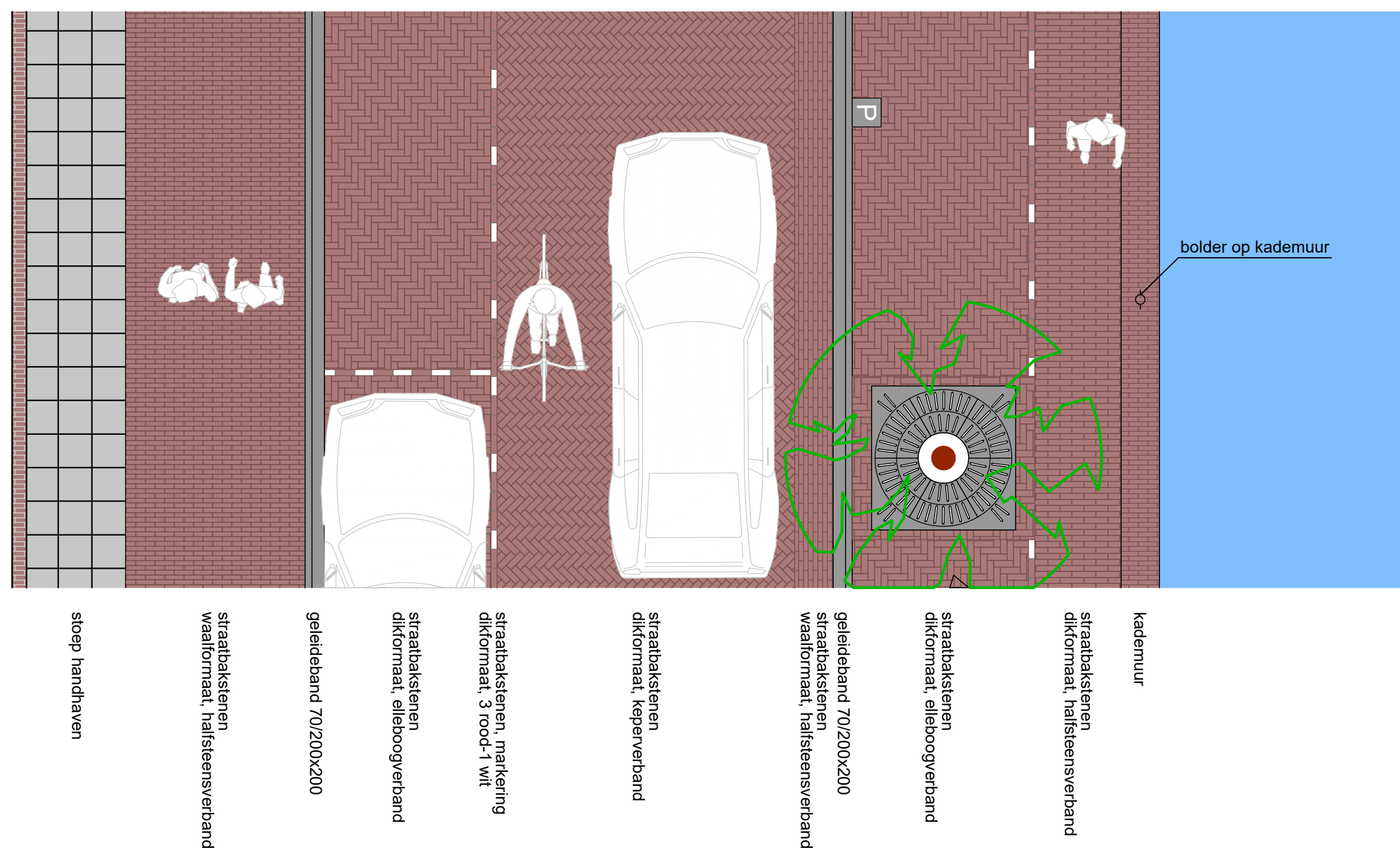
Principeprofiel A-A (2 zijden parkeren)
