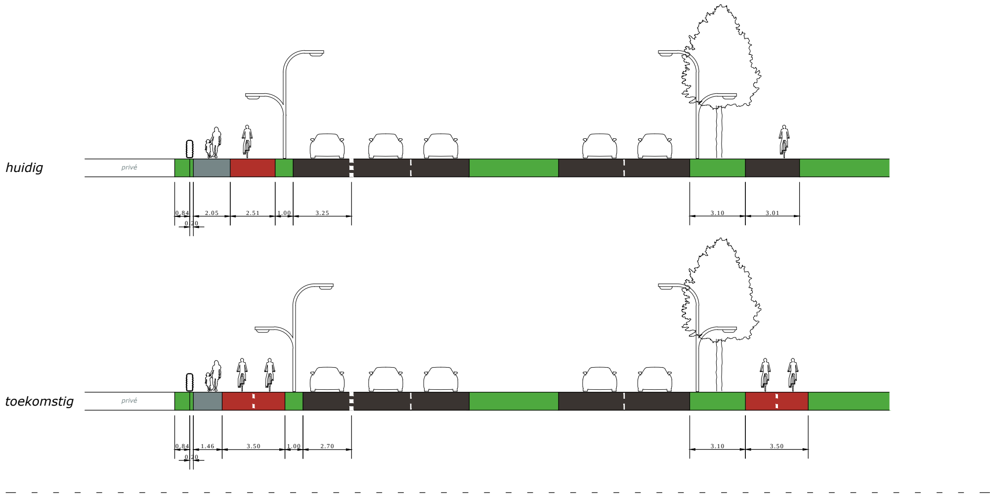
DWARSPROFIEL B
