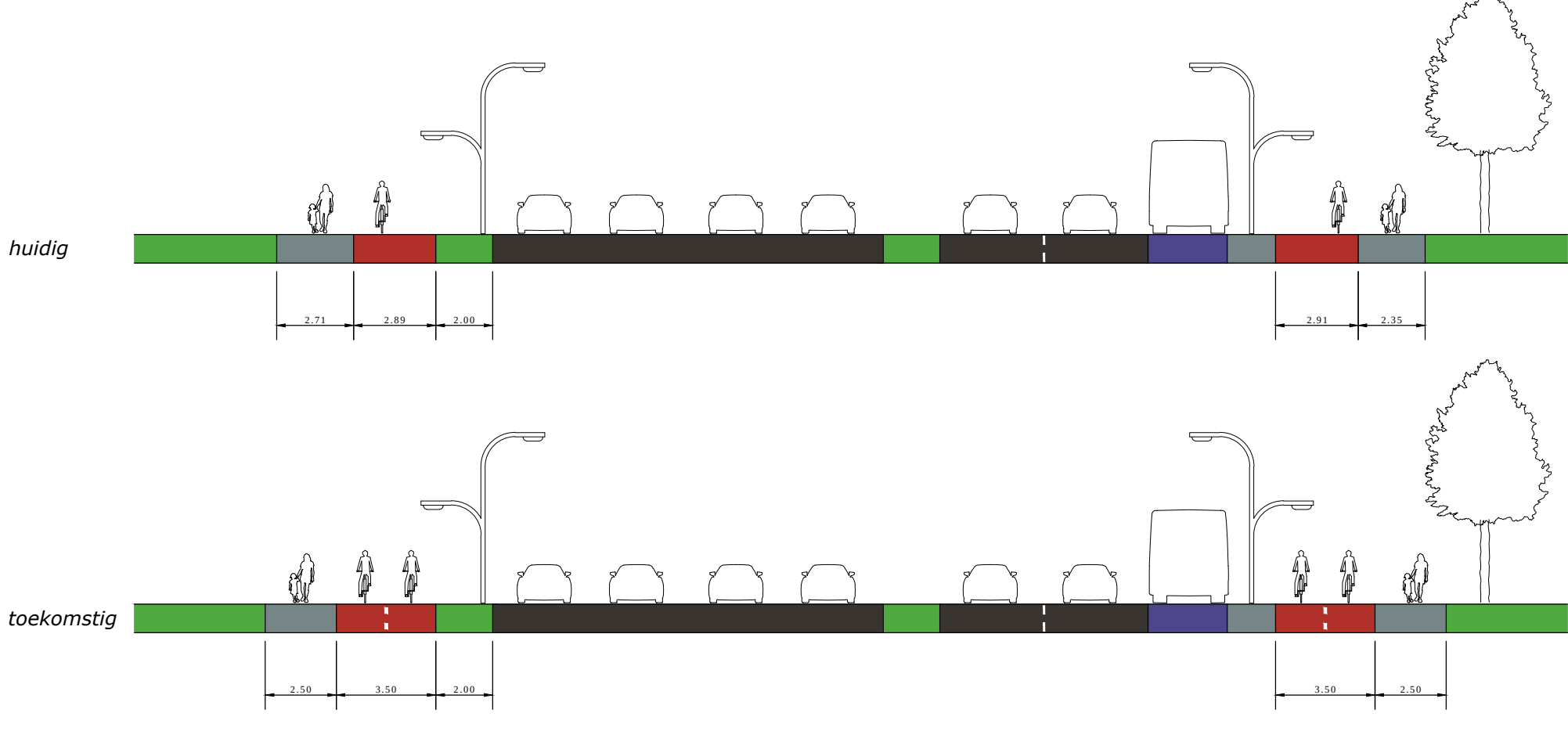
DWARSPROFIEL D
