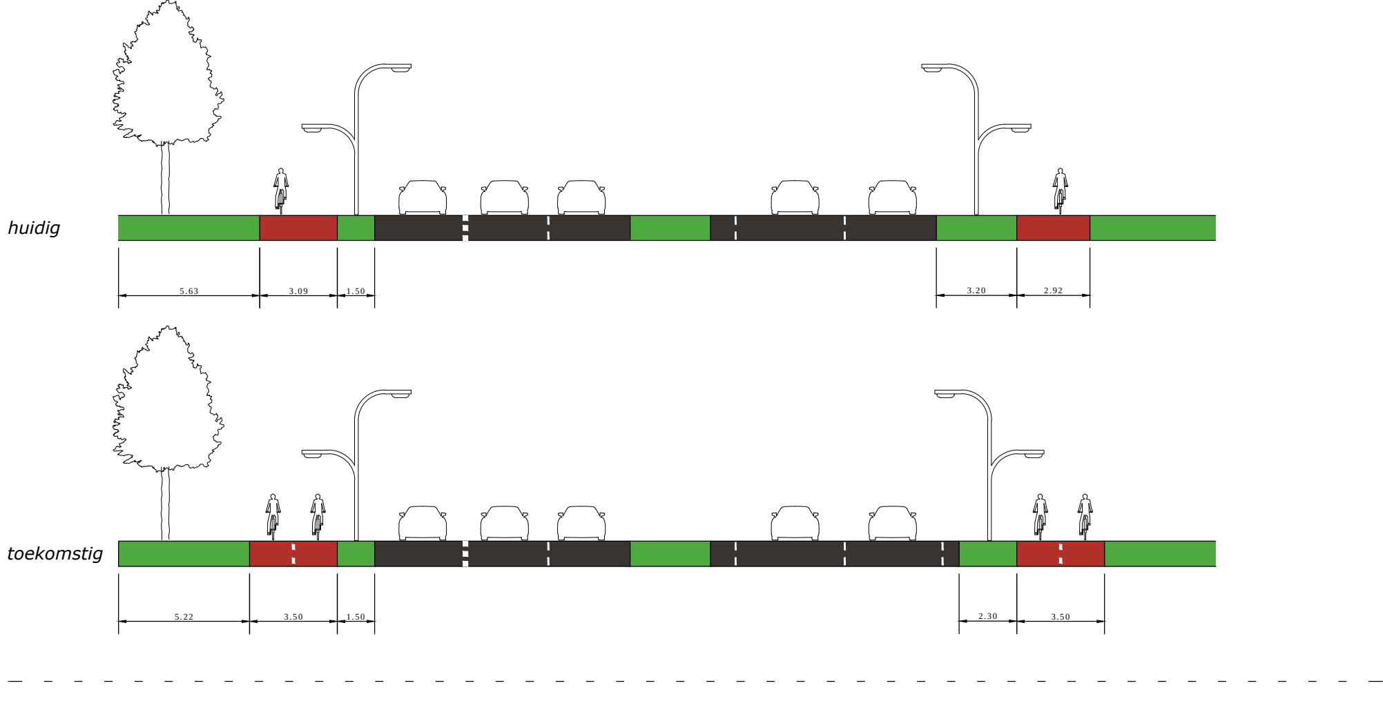
DWARSPROFIEL C
