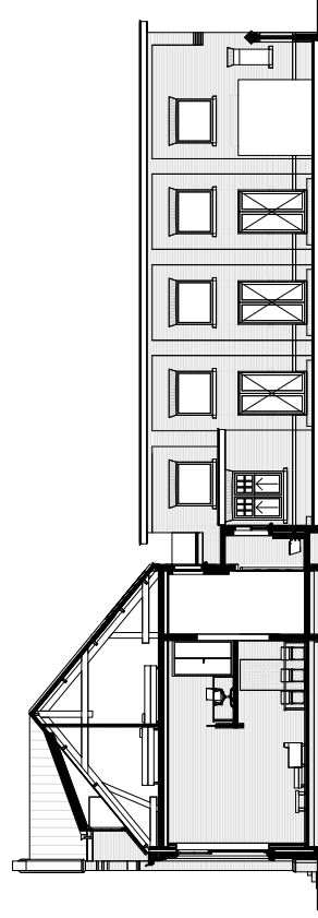
DOORSNEDE A-A (NIEUW)
