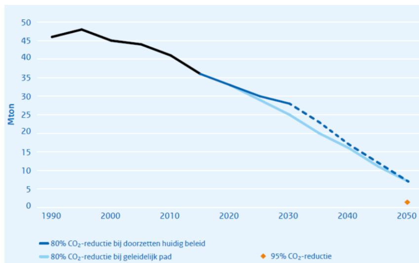
Figuur 7.1 Transitiepad CO 2 -uitstoot ruimteverwarming en tapwater (lage temperatuur warmte)
