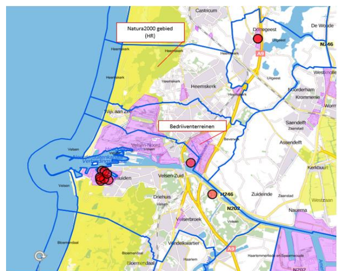
Figuur 5 - Ammoniakkoelinstallaties
