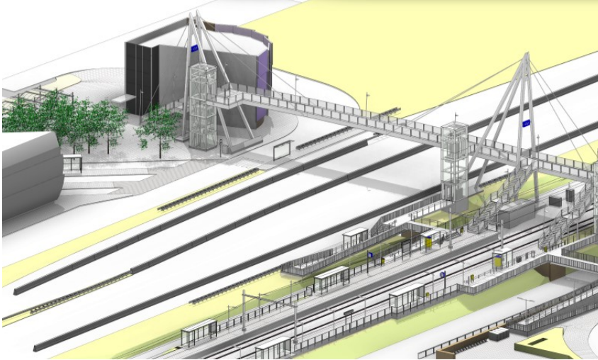
Ontwerp liften bij station Haarlem Spaarnwoude
