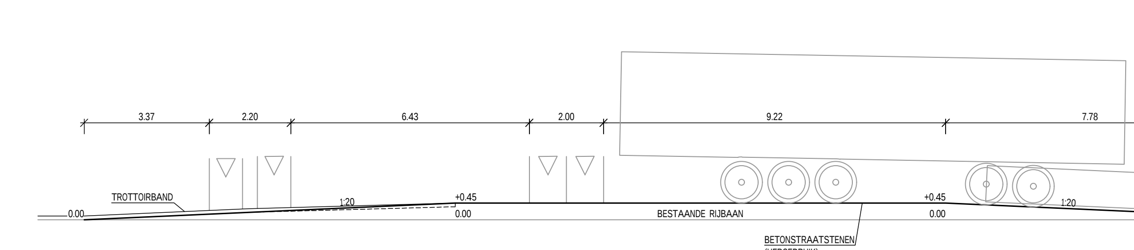
DWARSPROFIEL 3 SCHAAL 1:100
