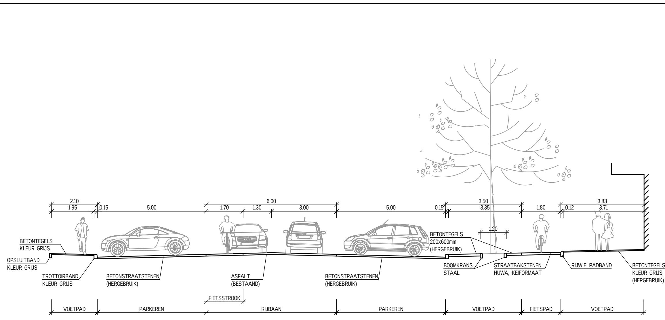
DWARSPROFIEL 1 SCHAAL 1:100
