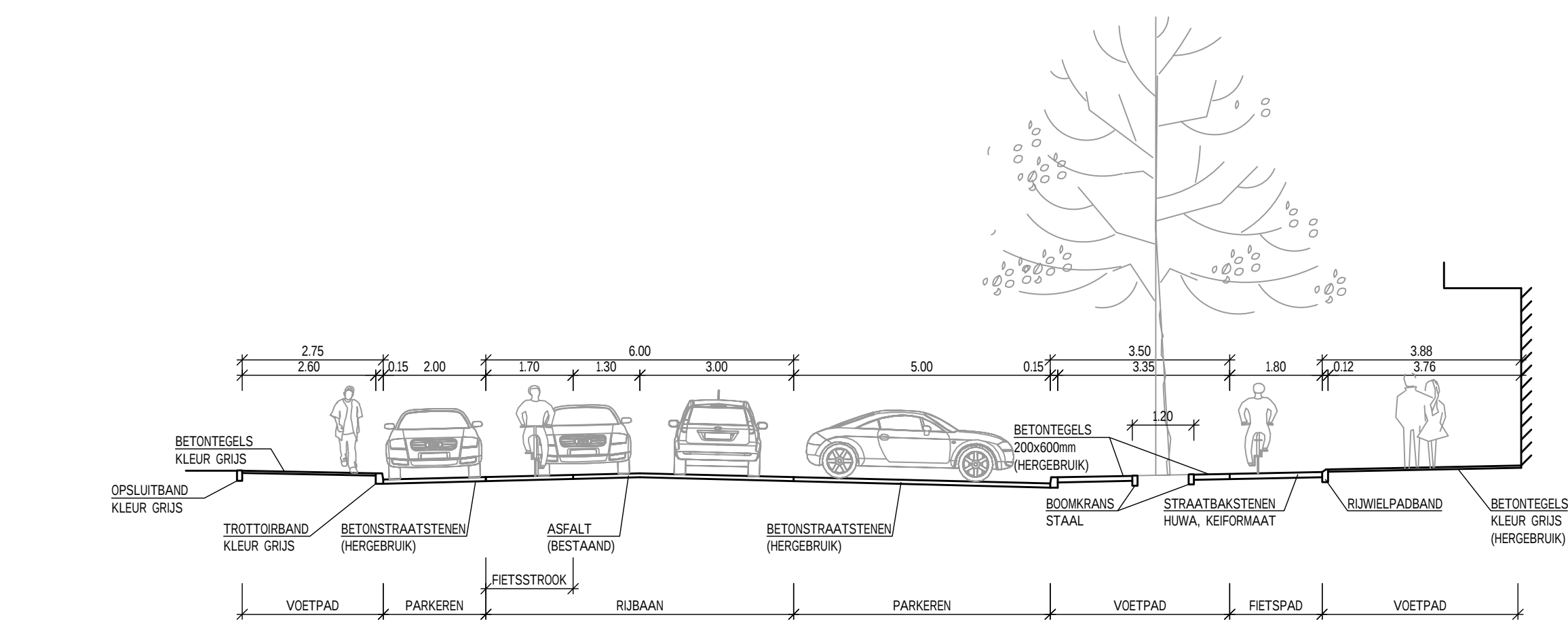
DWARSPROFIEL 2 SCHAAL 1:100
