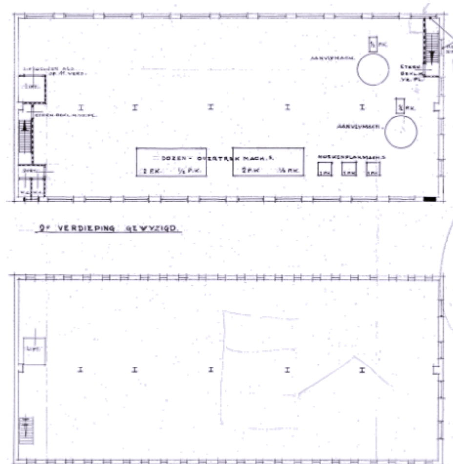
Plattegrond van de tweede verdieping met boven de nieuwe situatie en onder de bestaande situatie op de tekening van 1954. GABD.
