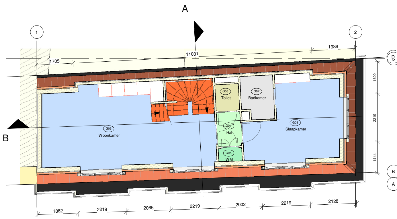
Derde verdieping (Nieuw) Schaal 1 : 100
