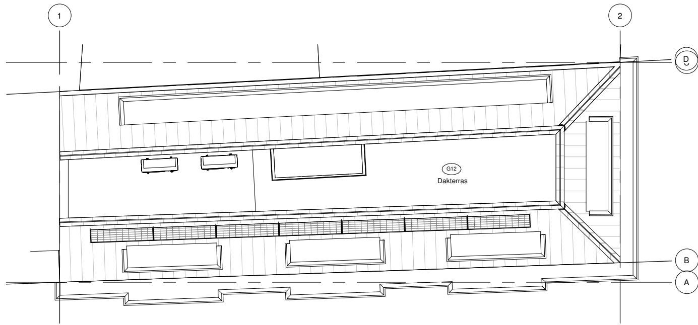
Dakaanzicht (Nieuw) Schaal 1 : 100
