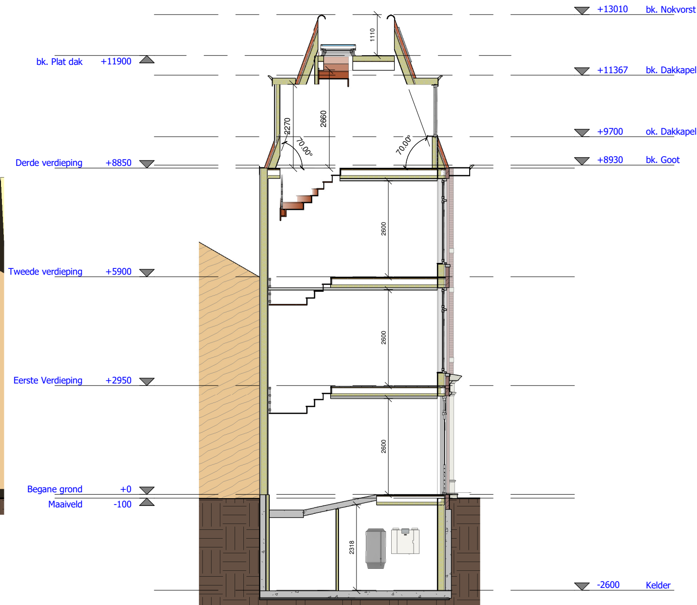
Doorsnede A-A (Nieuw) Schaal 1 : 100
