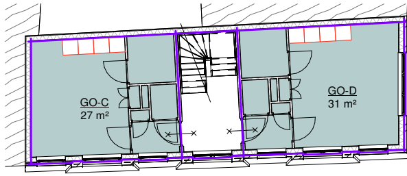
GO VD1 (Nieuw) Schaal 1 : 200
