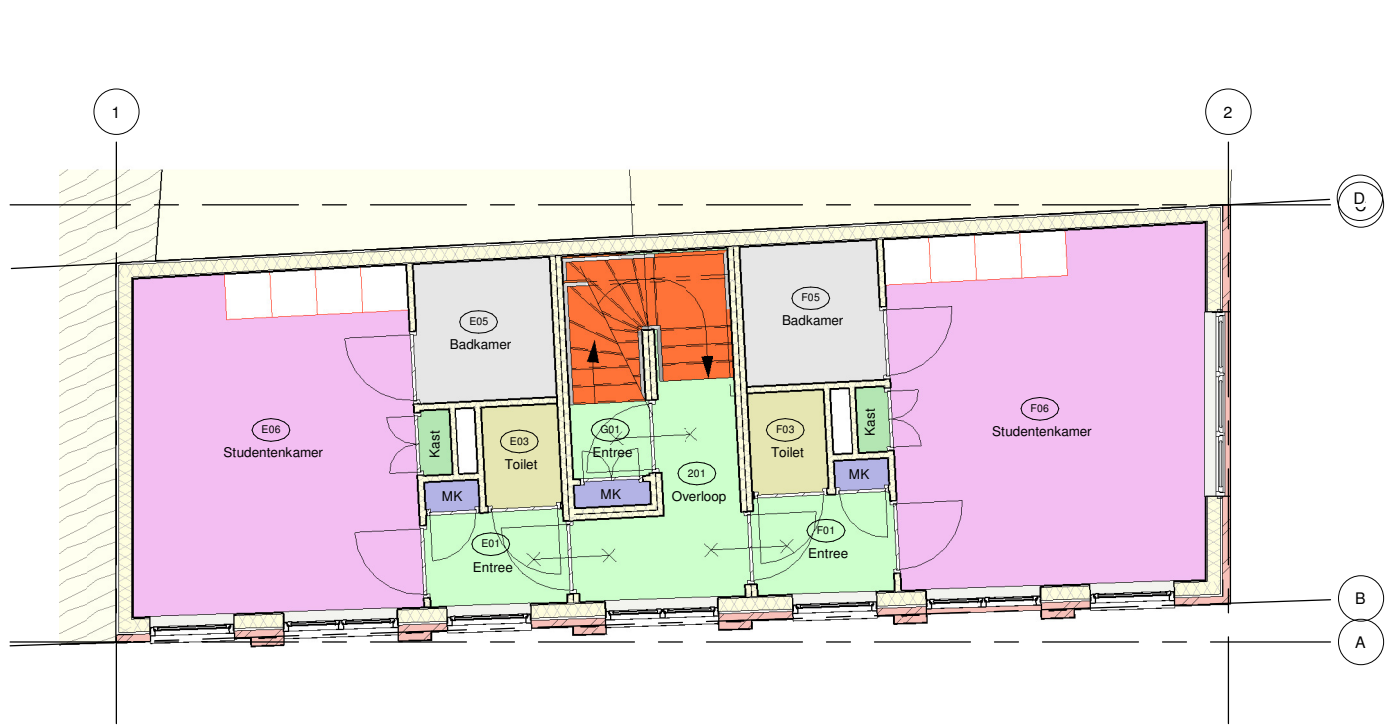
Tweede verdieping (Nieuw) Schaal 1 : 100
