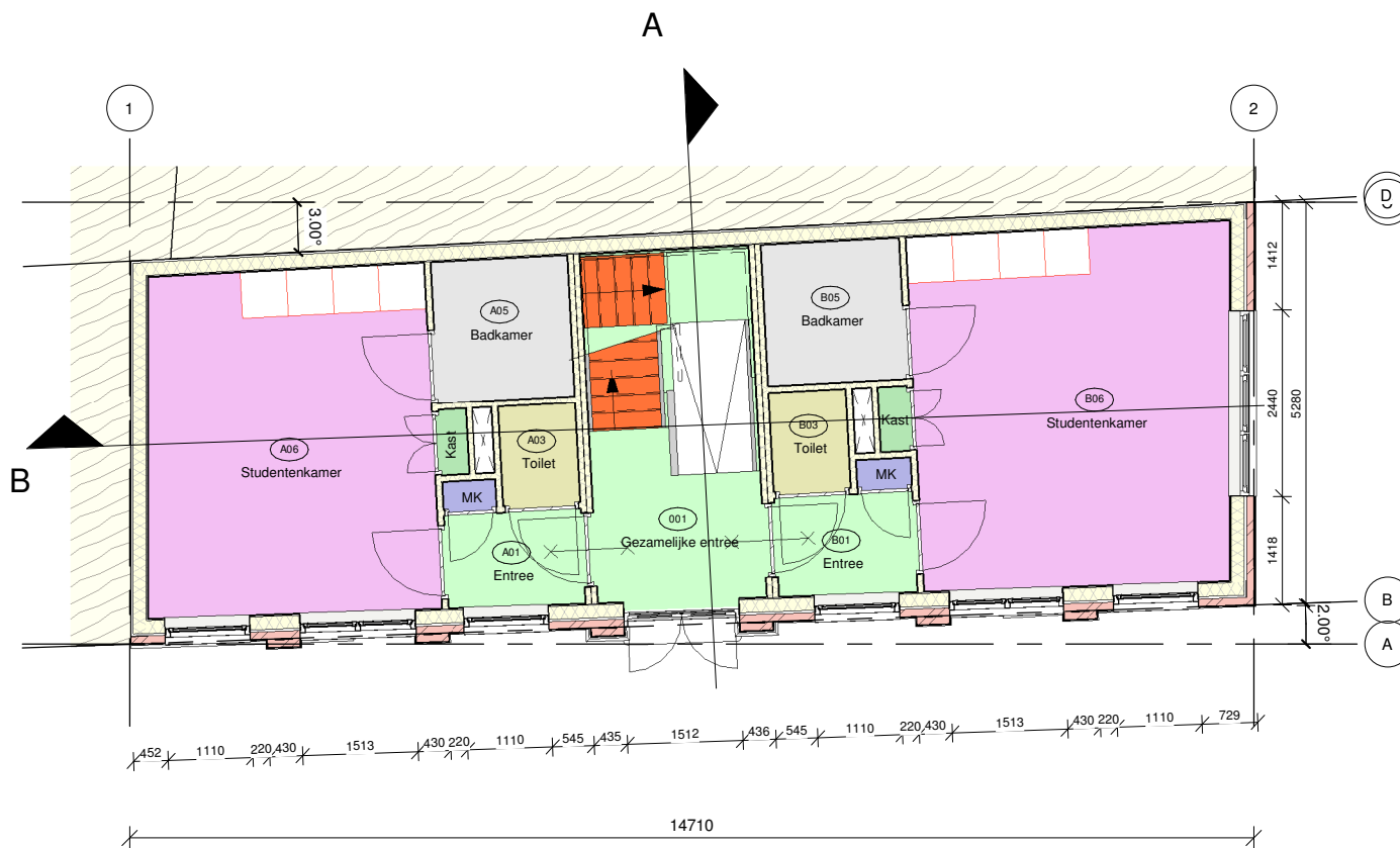
Begane grond (Nieuw) Schaal 1 : 100
