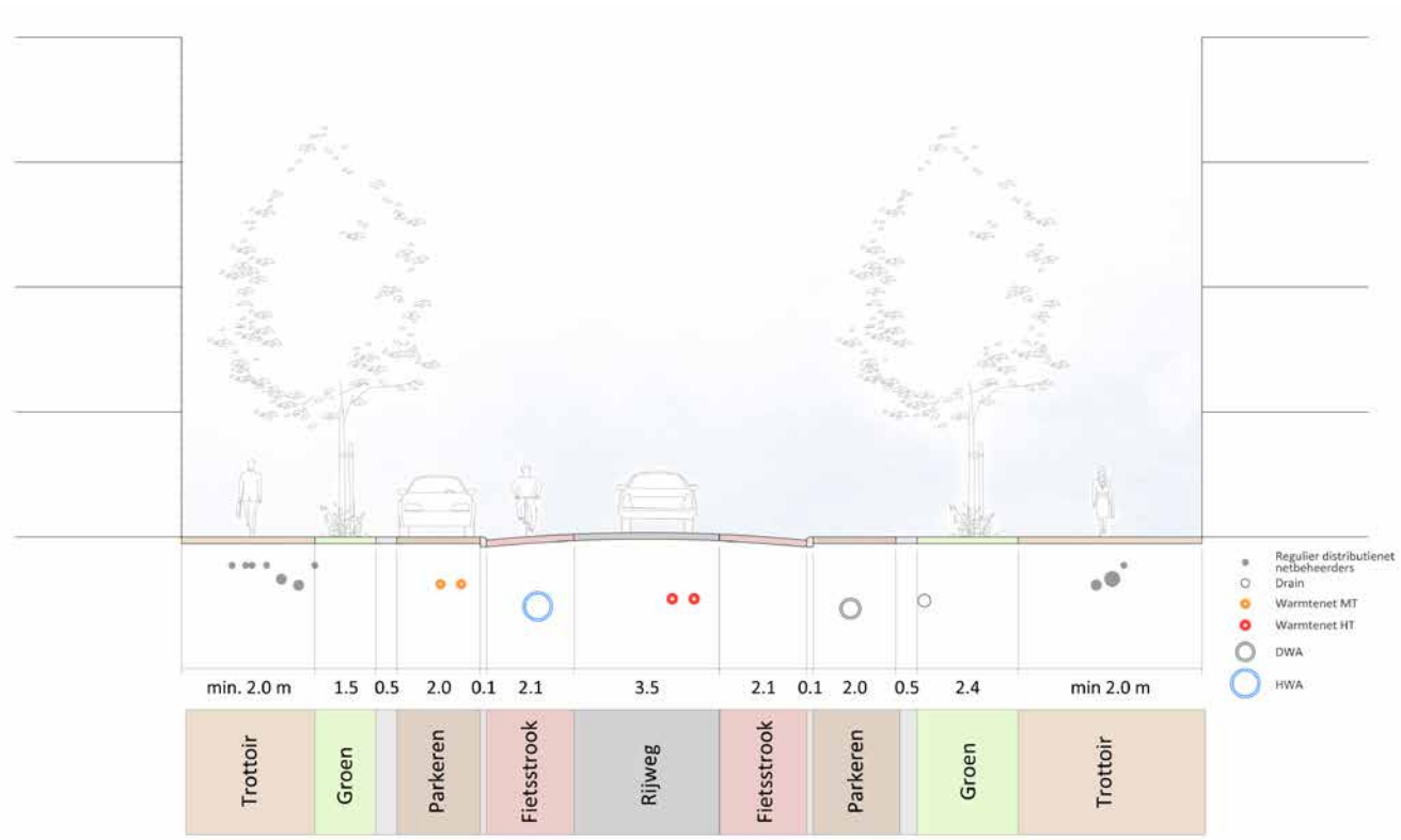
Standaard profiel buurtontsluitingsweg B
