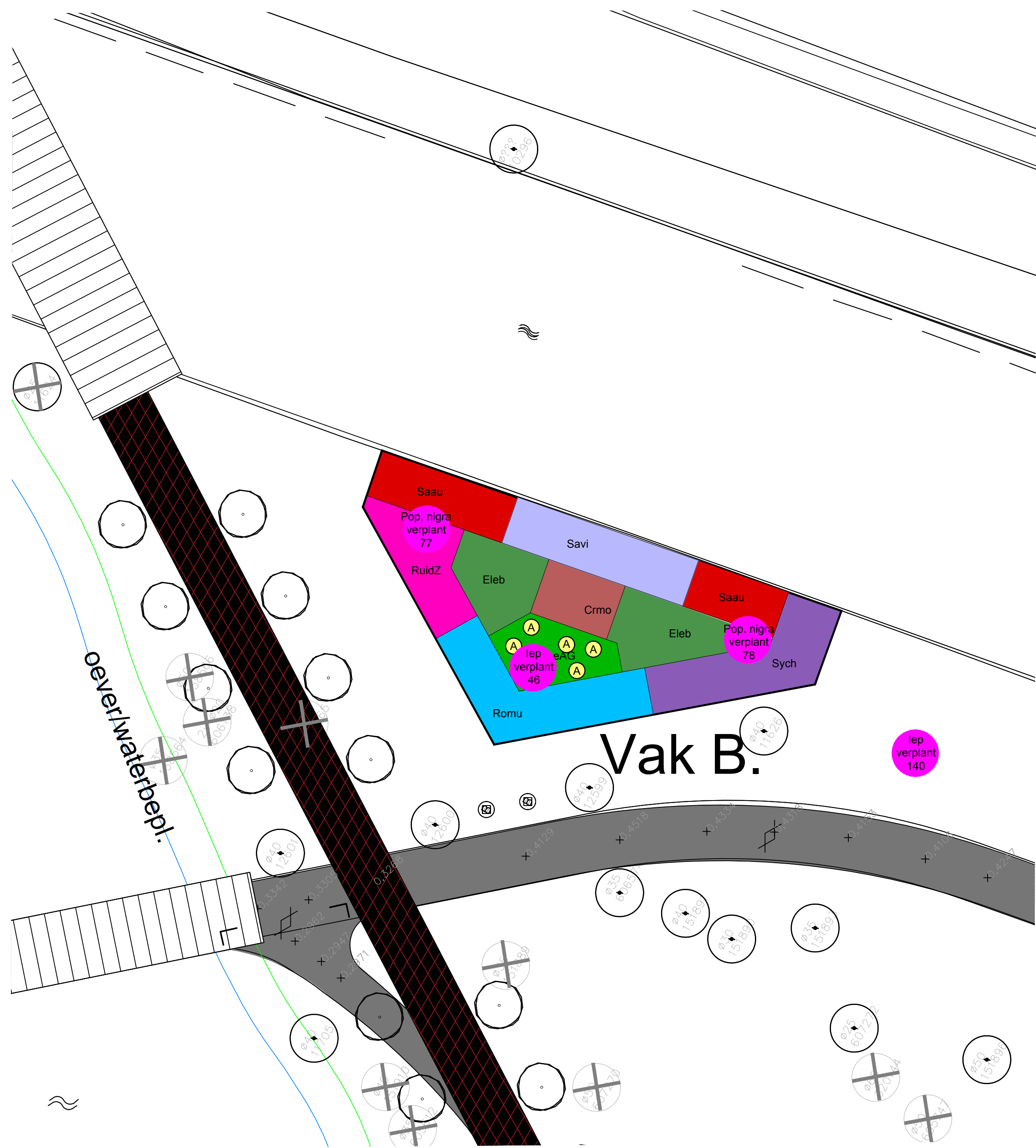
Bepantingsvak B schaal 1:200
