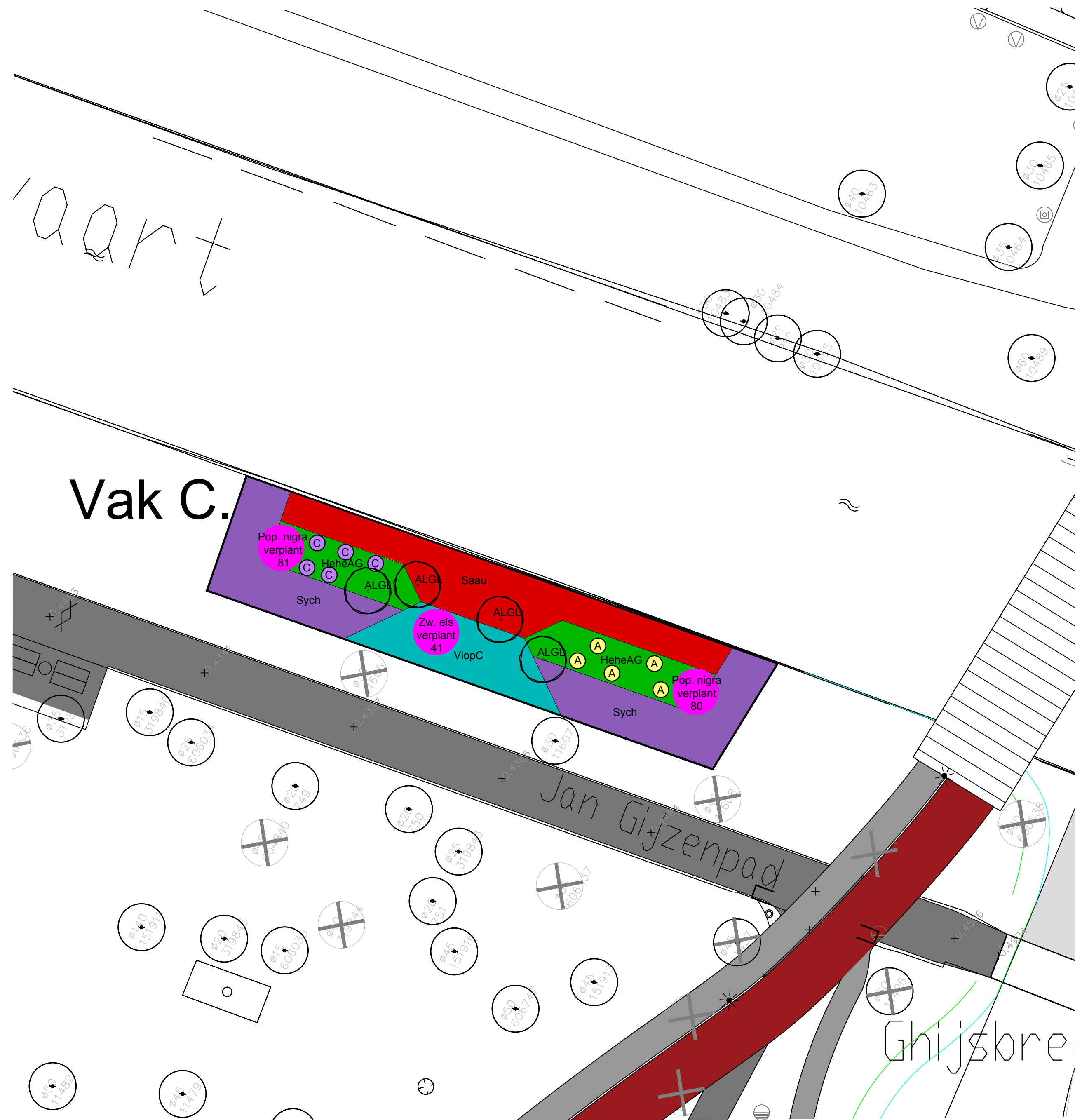
Bepantingsvak C schaal 1:200
