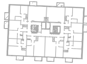
6e verdieping toren
