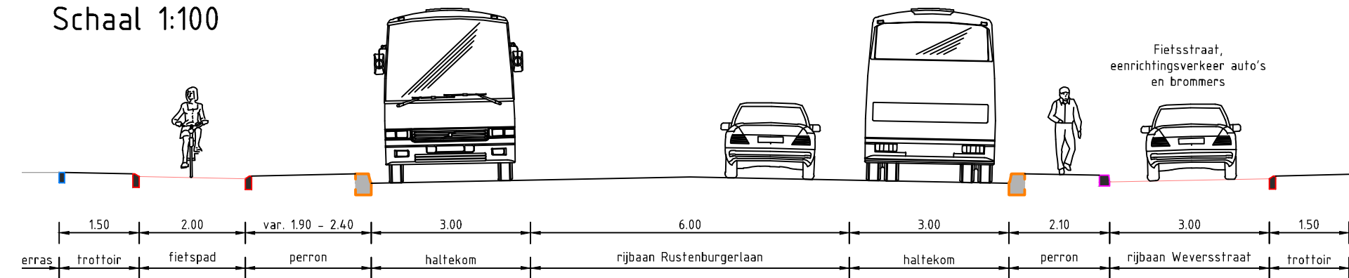
Principeprofiel Rustenburgerlaan (Doorsnede A-A) Schaal 1:100
