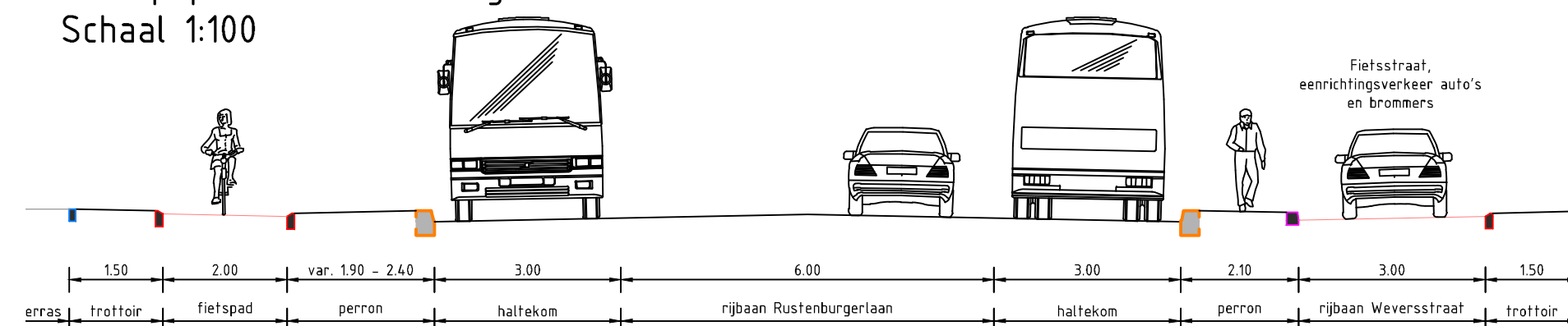
Principeprofiel Rustenburgerlaan (Doorsnede A-A) Schaal 1:100
