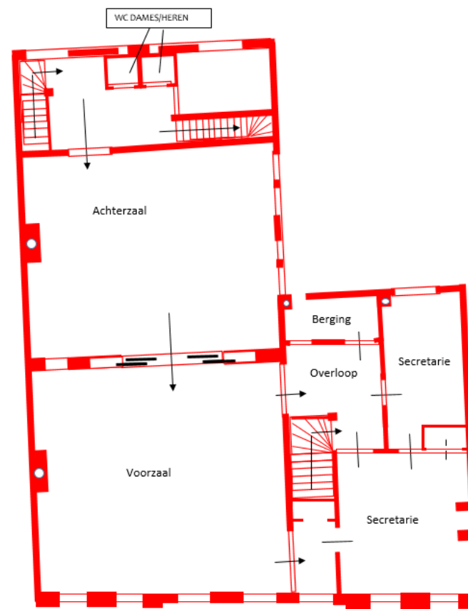
Reconstructie plattegrond verdieping, toestand 1887. FH MAB 2018
