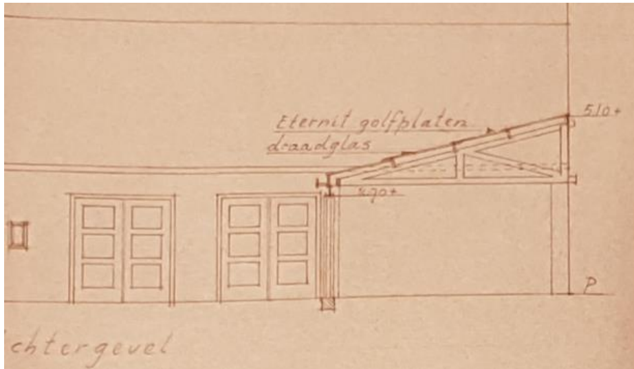
Achtergevel en doorsnede met nieuw lessenaardak over nieuwe stalling politie achter Lange Wijngaardstraat 12, nieuwe toestand. Dienst Openbare Werken Haarlem, dienstjaar 1949. NHA
