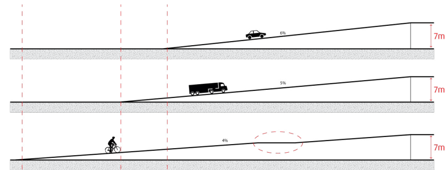
Indicatie benodigde lengte hellingbaan
