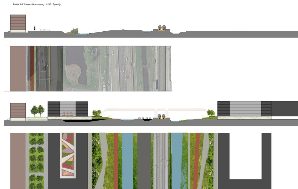
Mogelijke uitwerking nieuw profiel Amsterdamsevaart.
