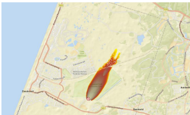
Figuur 5. Natuurbrandverspreiding 4 uur later na een mislukte eerste aanval. Vliegvlug slaat over de spoorlijn.
