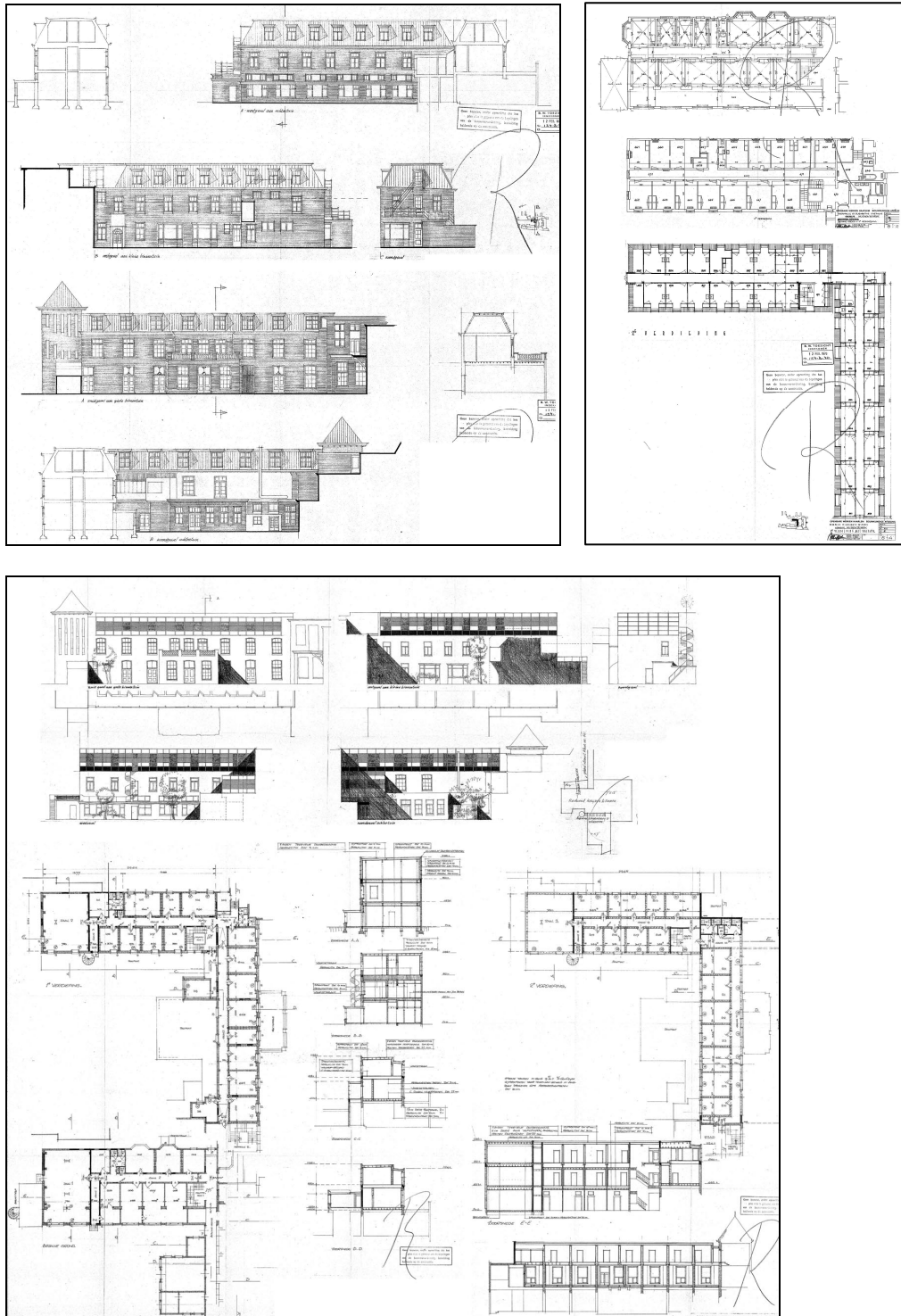
Afb. 18) Compilatie van tekeningen uit 1976 van de bestaande toestand (boven) en te maken toestand (onder) in de klasse- en zustervleugel. De verdiepingen van beide vleugels worden verbouwd ten behoeve van het Muziekcentrum Zuid-Kennemerland. De verbouwing is met name voor de zolderverdiepingen ingrijpend (rechts onder), die geheel worden herbouwd met vakwerkgevels. Bij de zustervleugel wordt aan de zuidzijde het beeld van 1905 gerespecteerd (afb. 4). (Herkomst: GH)
