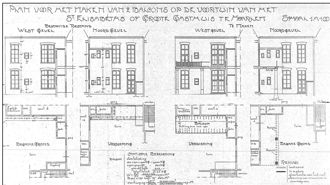
Afb. 8) Boven: plan uit 1924 voor het verbouwen van een eerste klas kamer op de verdieping van de regenten- en keukenvleugel tot kinderzaal. (Herkomst: GH)
