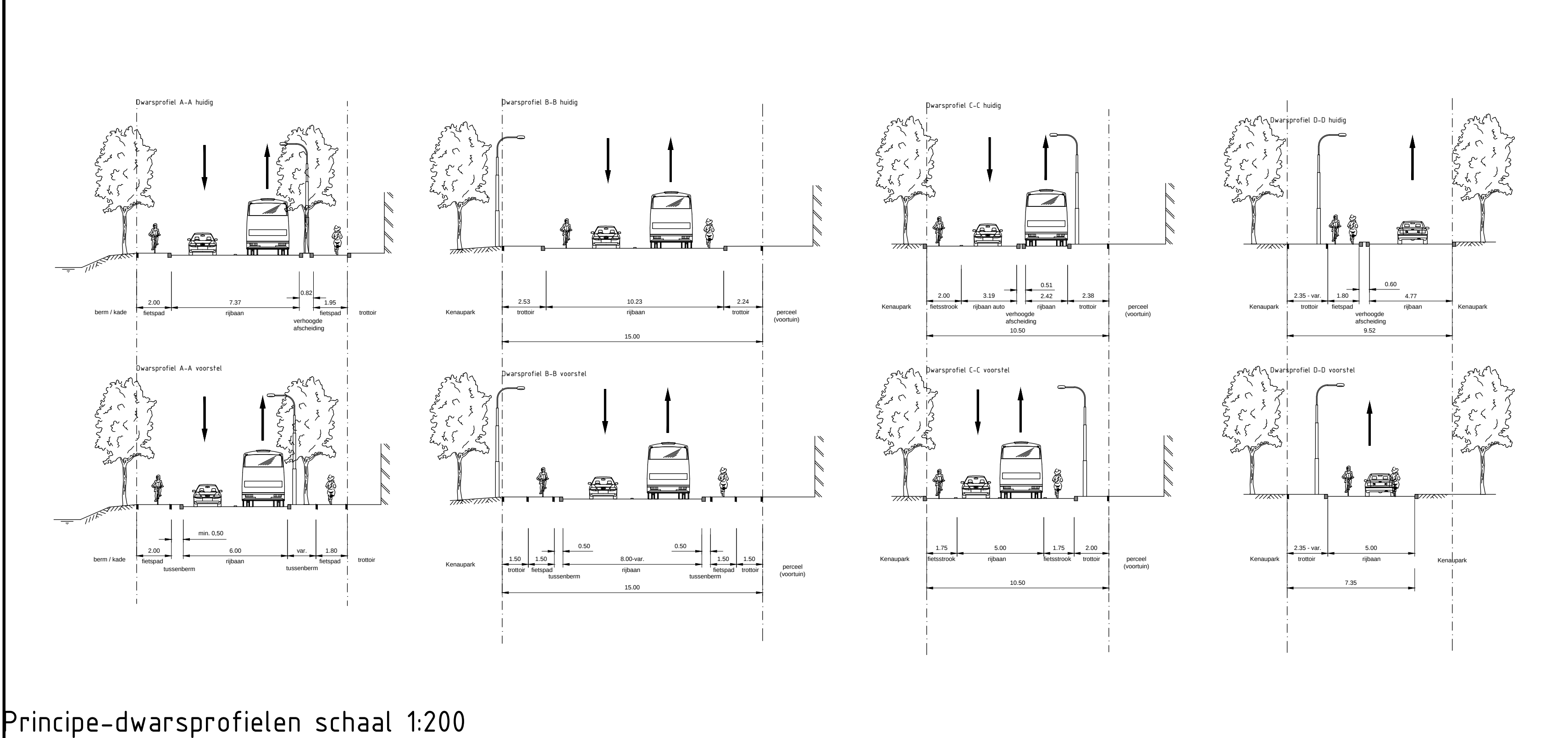
Principe-dwarsprofielen schaal 1:200
