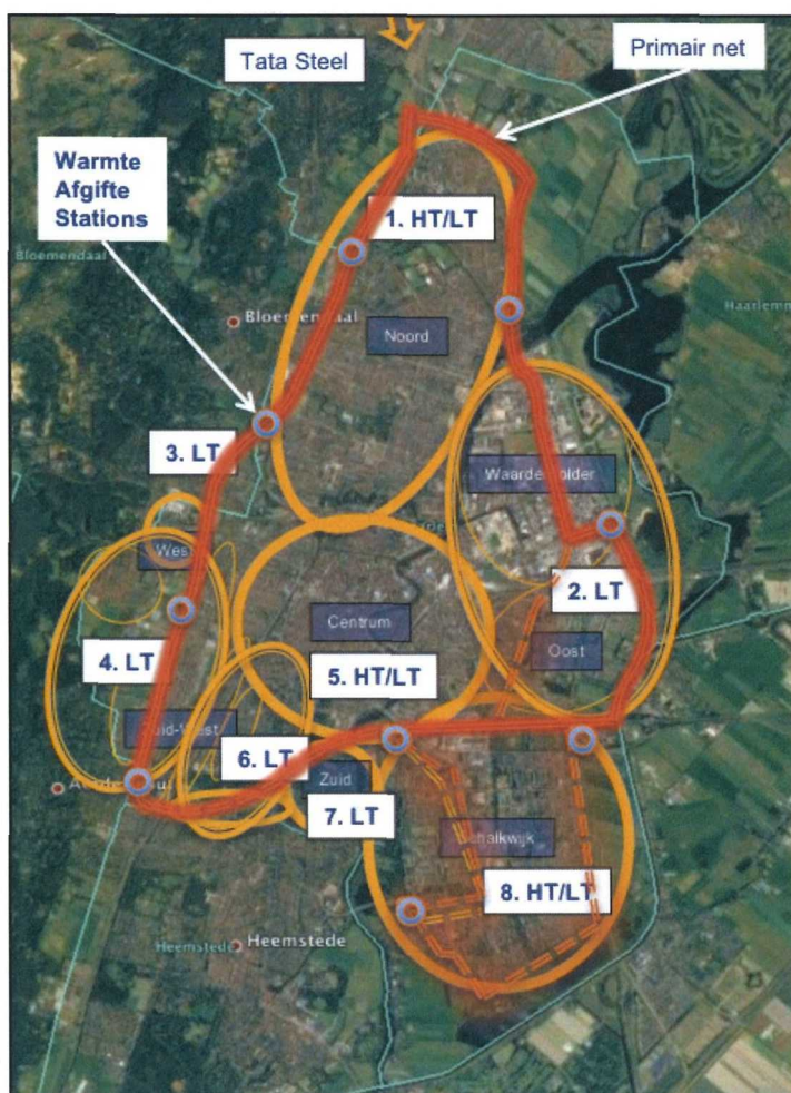
Samengesteld open hoge en lage temperatuurnetwerk
