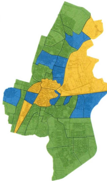
Figuur 10 Eindbeeld van de infrastructuur voor een klimaatneutrale warmtevoorziening in 2050. De aanname is dat alle energiedragers klimaatneutraal zijn in 2050
